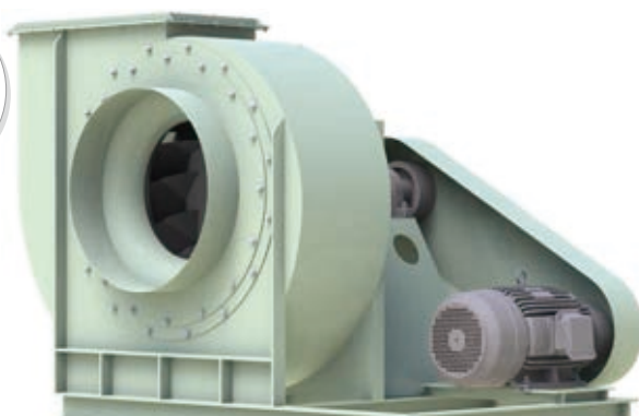
B55系列外觀示意圖
