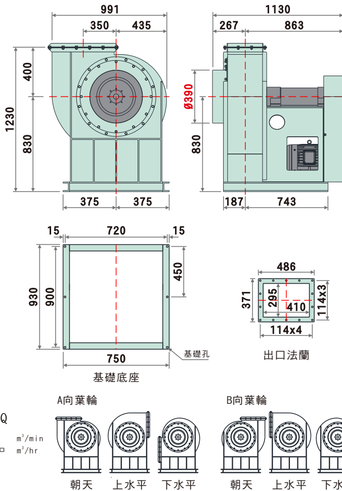
B55T系列外觀示意圖 B55T SERIES IMAGE
