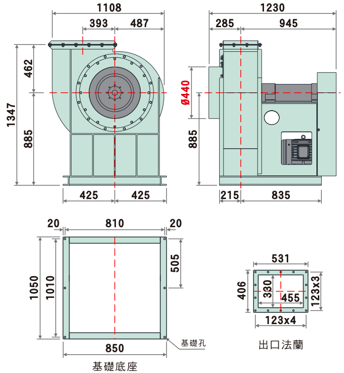
B55T系列外觀示意圖 B55T SERIES IMAGE
