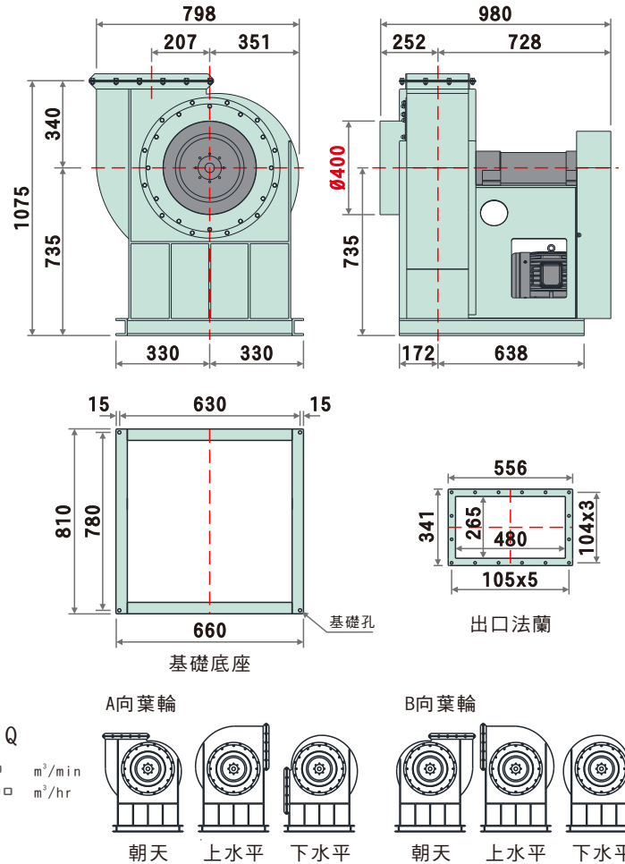
B59系列外觀示意圖 B59 SERIES IMAGE
