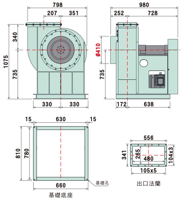
A向葉輪
